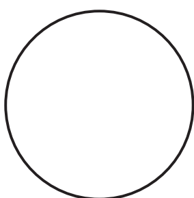
Llena
