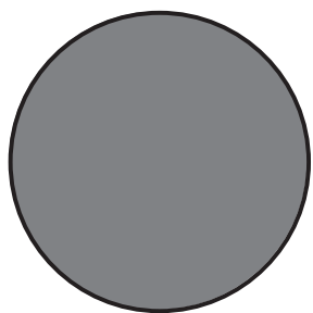
Nueva
