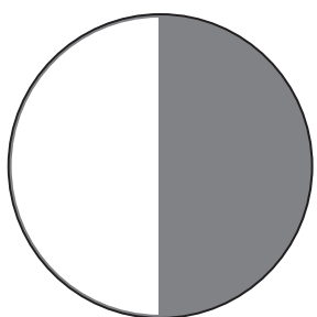
Cuarto menguante
