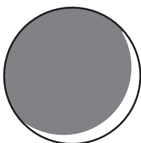
Creciente
