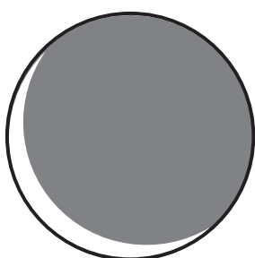
Menguante
