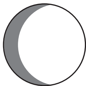
Creciente gibosa
