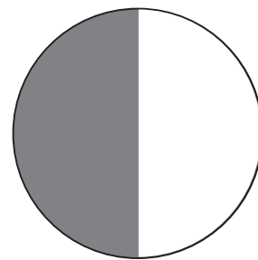
Cuarto creciente
