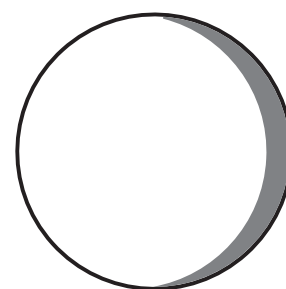
Menguante gibosa
